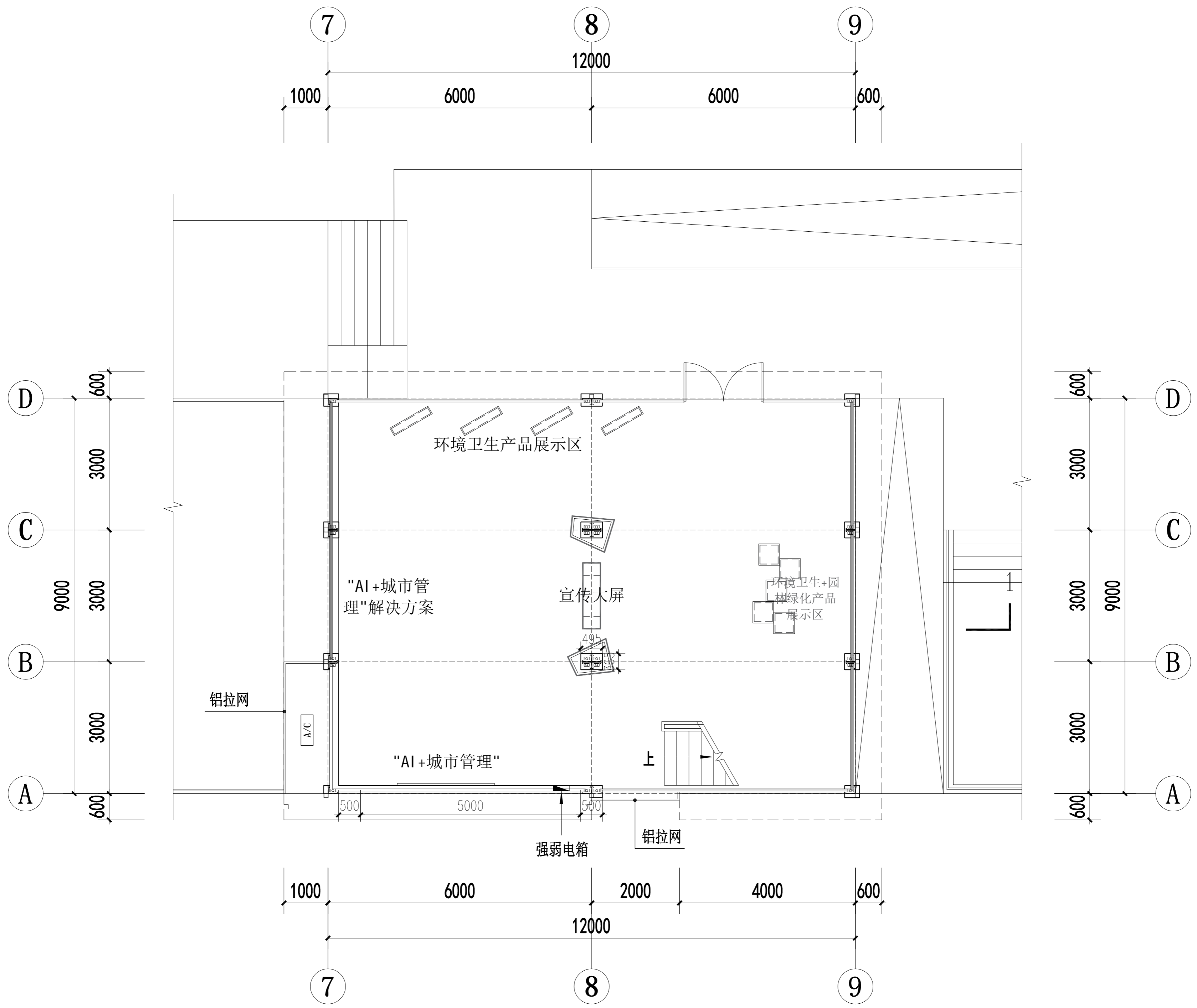
C栋一层平面图 (108m 2 )
