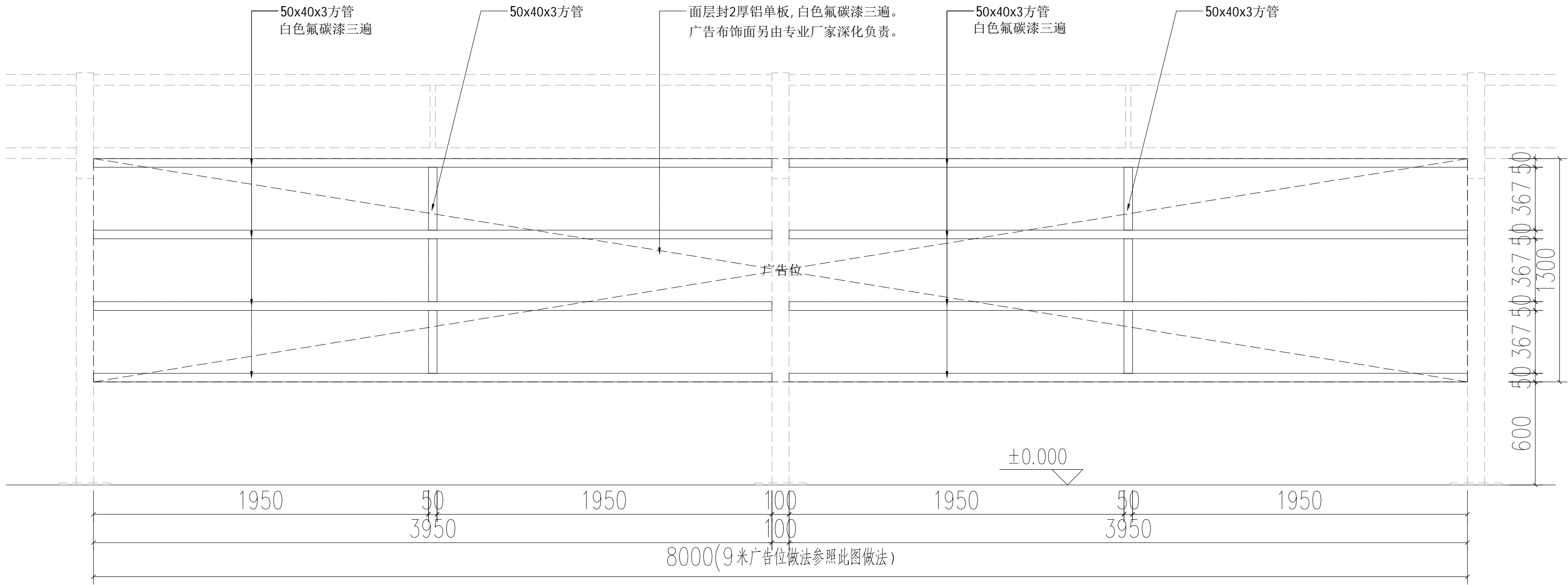
KEY PLAN 广告布结构单元立面图 SCALE 1:30 @A2
