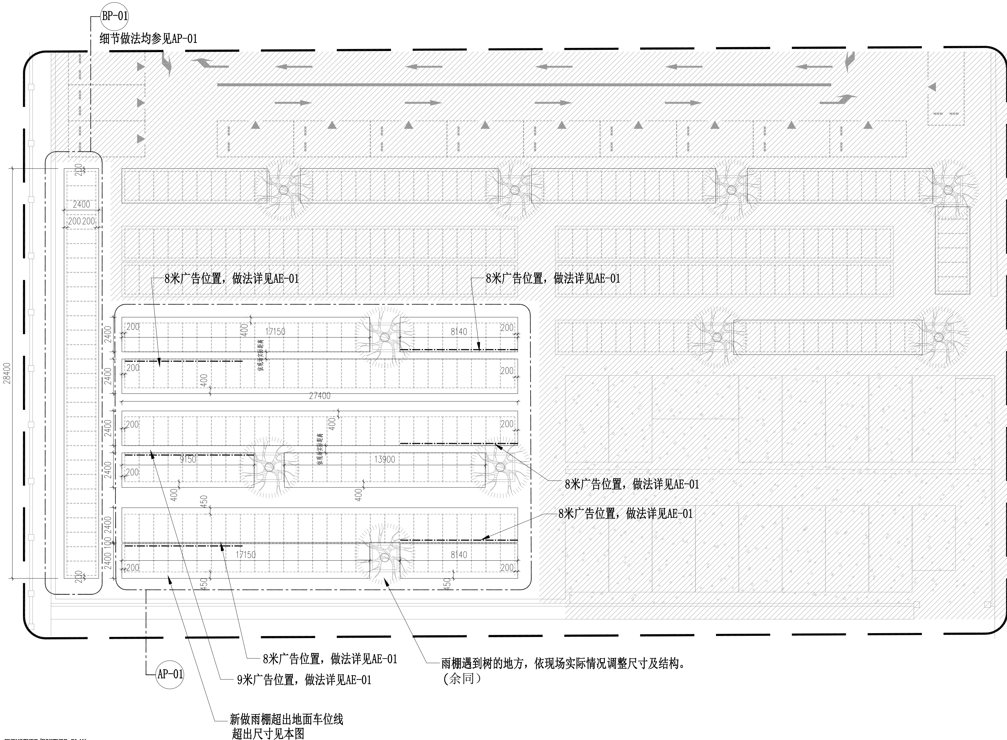
FURNITURE/FIXTURE PLAN 平面布置图 SCALE 1:150 @A2
