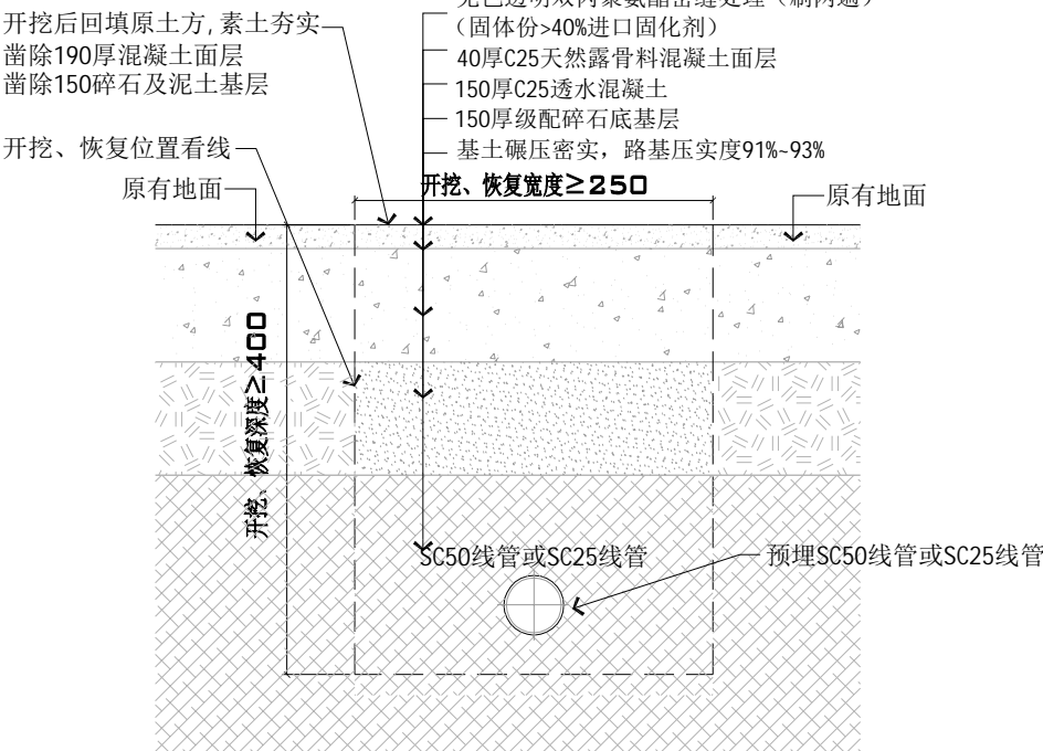
地面埋管开挖恢复示意图
