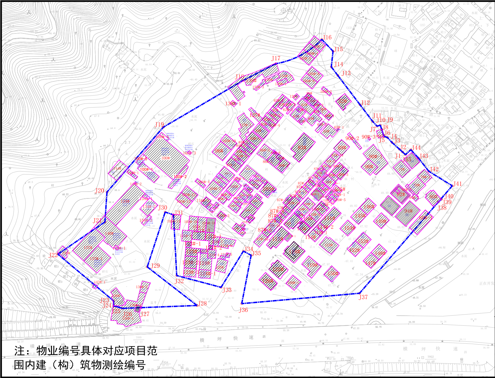
附件1: 龙岗区园山街道大福旧村城市更新单元一期拆除范围线及建筑物权属分布图
